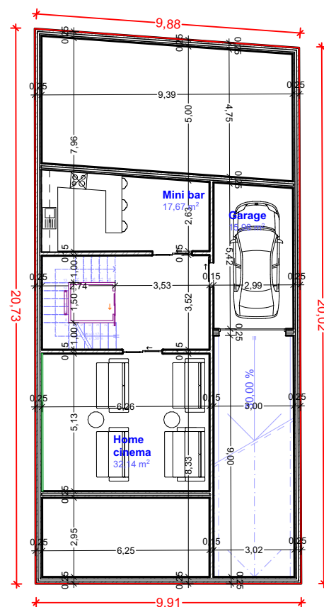
Plan sous-sol
