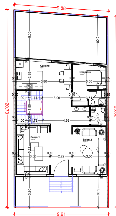
Plan RDC
